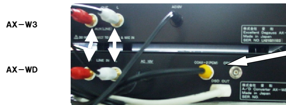
3図(AX-W3とAX-WDの接続)
